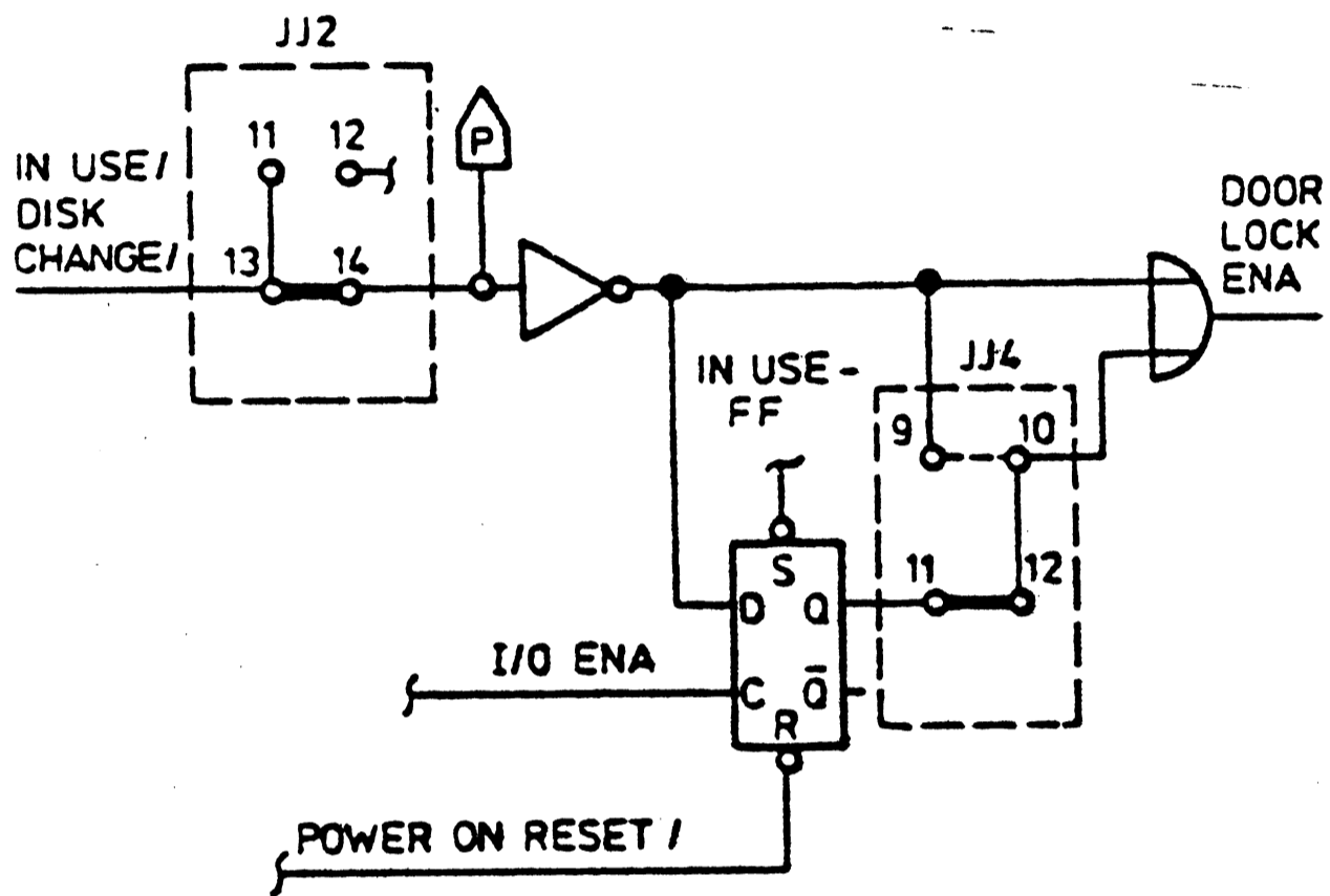
FIG. 2 - 13 DOOR LOCK OPTION
