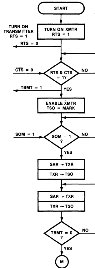
Fig. 12a BCP Transmit
