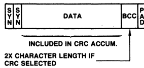
Fig. 9 BCP Message Format
