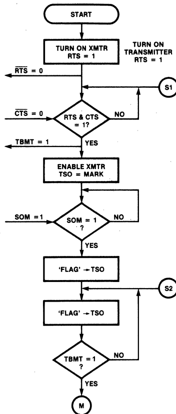
Fig. 10a BOP Transmit
