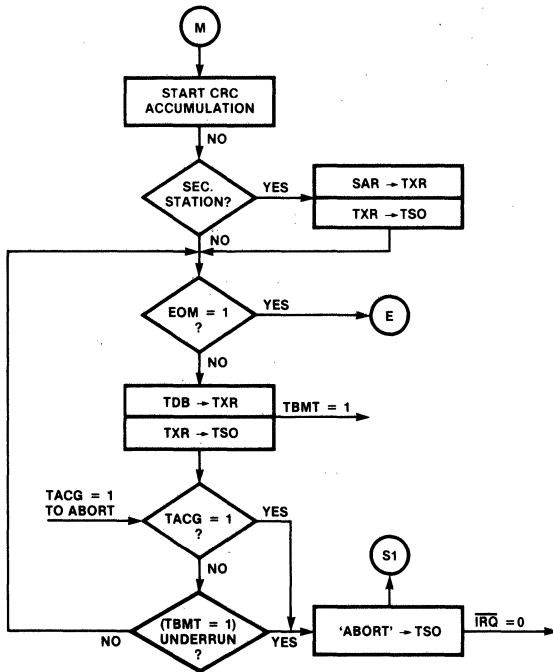
Fig. 10b BOP Transmit
