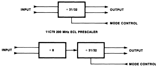
Fig. 19 Prescalers
