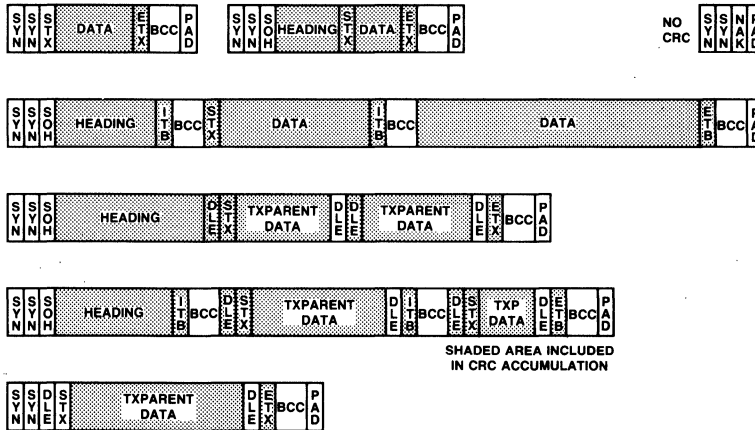
Fig. 7 BISYNC Message Format
