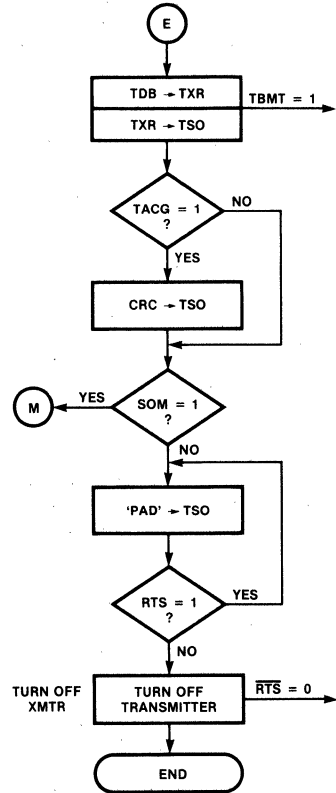
Fig. 12c BCP Transmit
