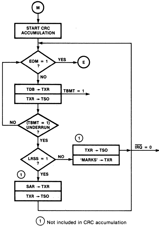
Fig. 12b BCP Transmit
